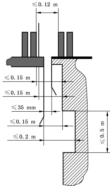
图 6 运载装置与面对运载装置入口的井道壁的间隙
