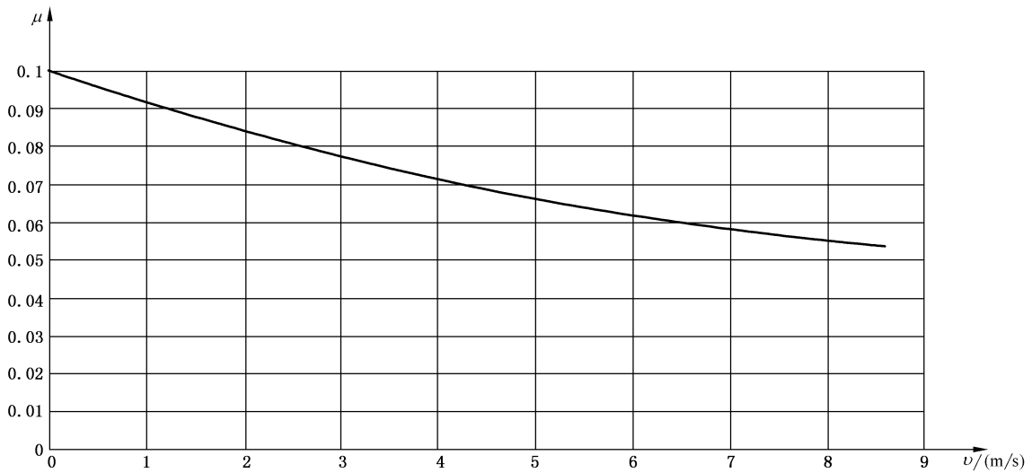
图 K.3 最小的摩擦系数
