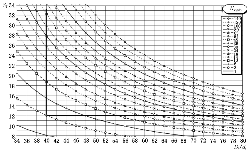
图 L.1 最小安全系数的计算
