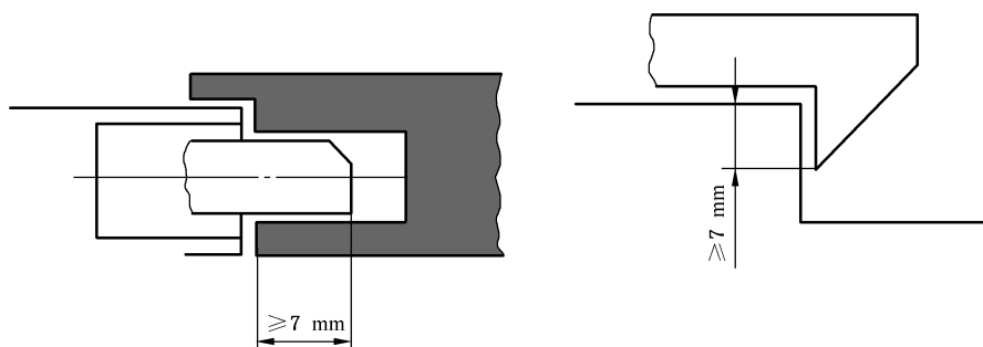
图 4 锁紧部件示例
