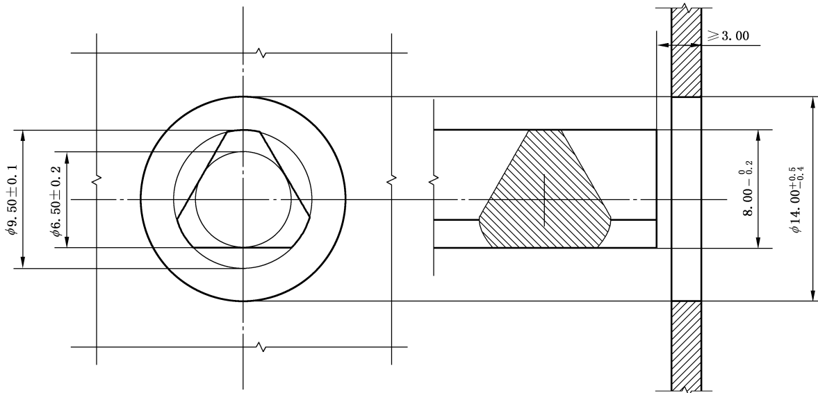
图 B.1 三角形开锁装置
