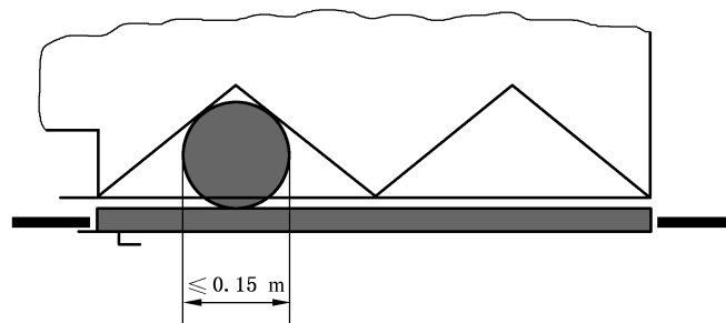
图 7 铰链层门和折叠运载装置门的间隙
